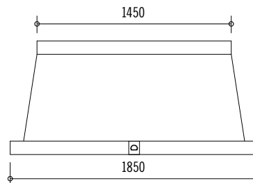
HOTTE CHÂTEAU 165 : H18T0
